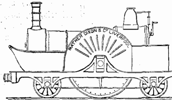
Фиг. 68. Паровозъ „Аѣах“ съ діаметромъ ведущихъ колесъ въ 10 футовъ, завода Mather, Dixon & Co.
