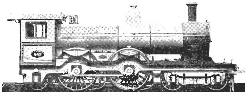
Фиг. 293. Пассажирскій паровозъ Голландской ж. д.
