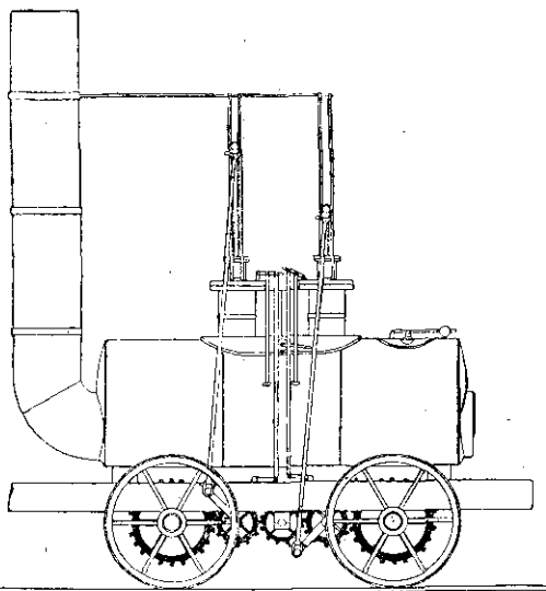
Фиг. 9. Первый паровозъ Георга Стефенсона „Блюхеръ“.
