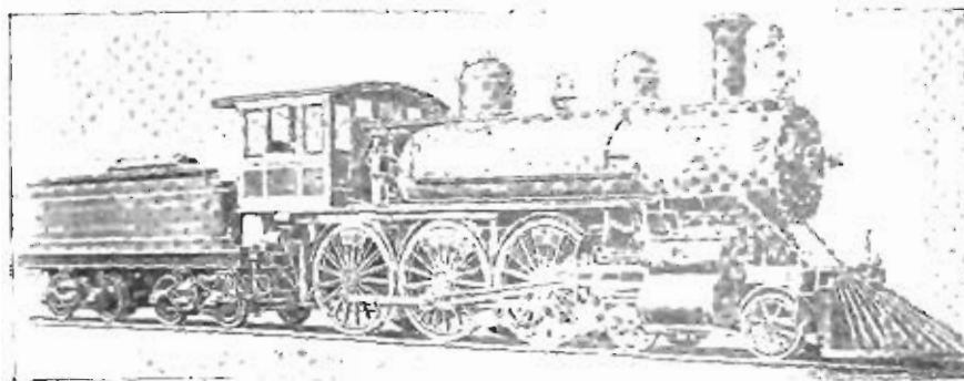
Фиг. 209. Паровозъ компаундъ системы Воклепа 1889 г.
