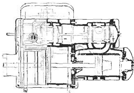
Фиг. 326. Устройство золотниковъ паровоза тендеръ-компаундъ завода Шенектади, 1900 г.
