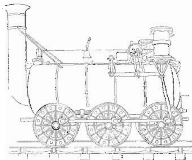
Фиг. 17. Паровозъ „Royal George“ Стоктонь-Дарлингтонской ж. д. 1827 г.
