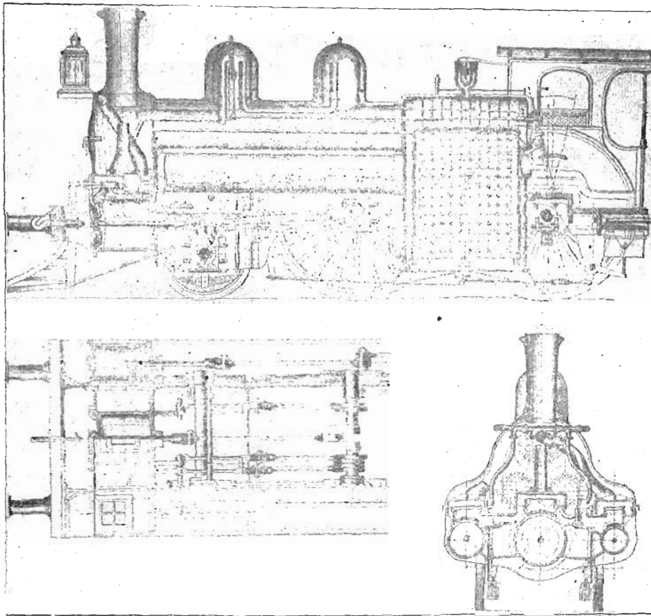
Фиг. 221-223. Паровозъ съ тройнымъ расширеніемъ пара.
