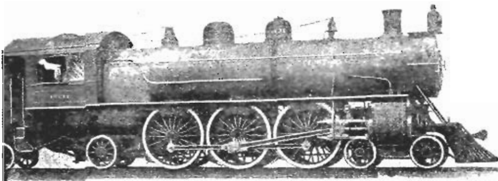
Фиг. 384. Паровозъ, построенный заводомъ Балдвина для жел. дор. Chicago-Mon. 1903 г.
