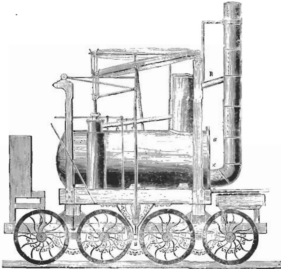
Фиг. 8. Паровозъ „Пыхтящій Вилли“, передѣланный въ 1813 г.
