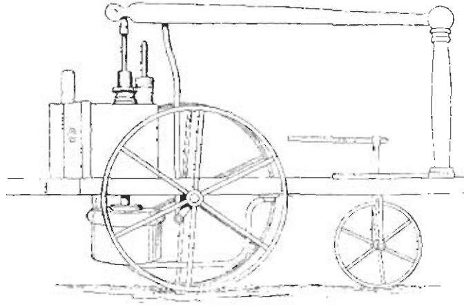
Фиг. 2. Паровозъ Murdoch'a.
