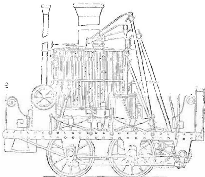
Фиг. 56. Паровозъ Джелингема и Уайнса Балтимора-Огайской ж. д. 1835 г.
