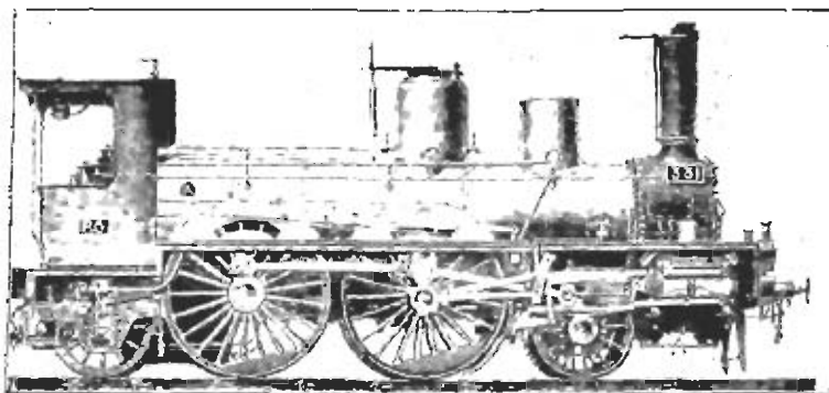
Фиг. 239. Паровозъ Парижъ-орлеанской жел. дороги съ парораспределеніемъ Polonceau.
