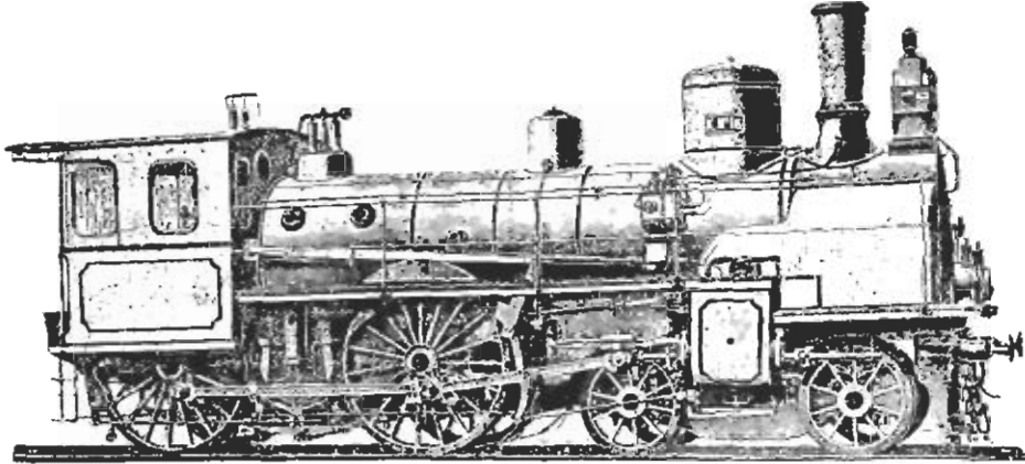
Фиг. 219. Пассажирскій двухцилиндровый compound паровозъ С.-Петербургско-варшавской жел. дор.
