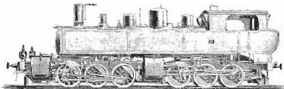
Фиг. 218. Паровозъ дуликель-компаундъ завода Маффая.
