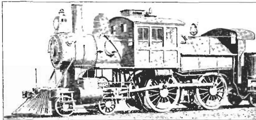
Фиг. 235. Паровозъ завода Кука 1893 года.
