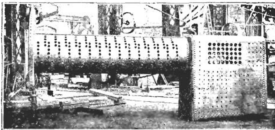
Фиг. 338. Водогрубный паровой котелъ. Внутренняя цилиндрическая часть и огневая коробка, съ отверстіемъ для поперечныхъ цилиндрическихъ трубъ.
