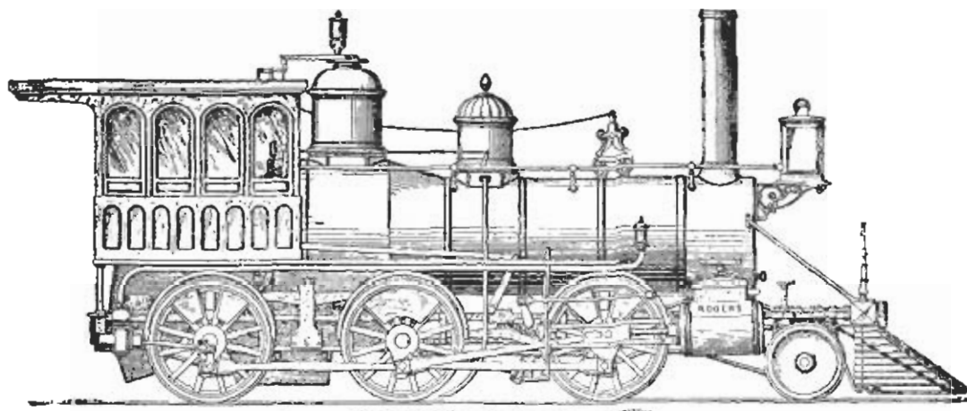
Фиг. 147. Первый паровозъ системы „Mogul“. 1863 г.
