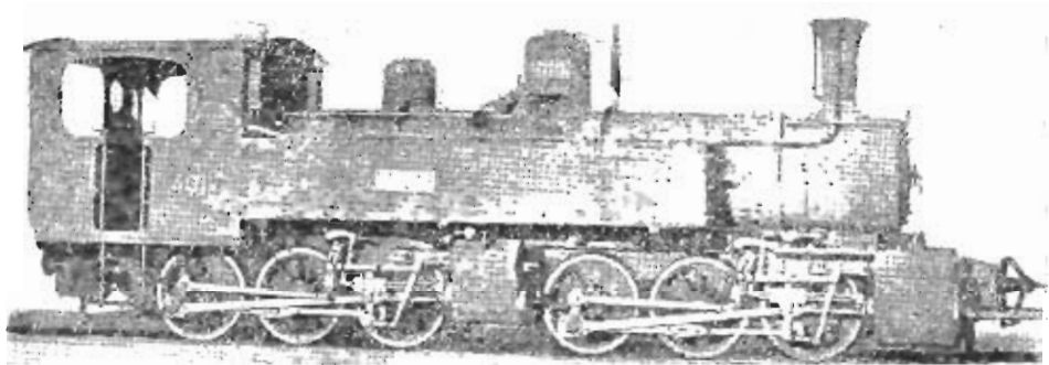
Фиг. 372. Танковый паровозъ дулкесъ-компаундъ системы Маллета. 1903 г.
