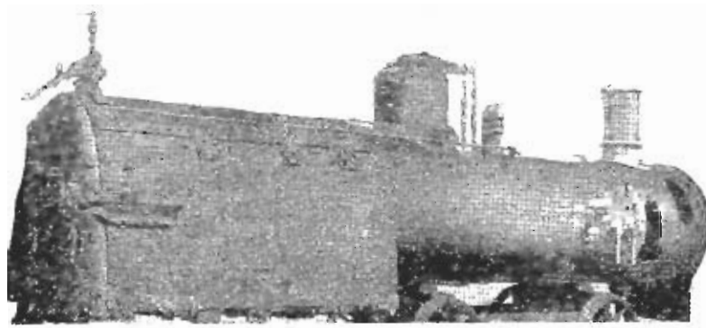
Фиг. 380. Водяной котелъ.
