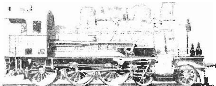
Фиг. 378. Пассажирскій паровозъ типа 1 австрійской Северо-Южной ж. д. 1903 г.
