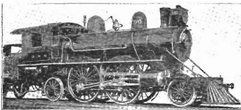
Фиг. 254. Пассажирскій паровозъ типа „Columbia“ завода Бальдина.
