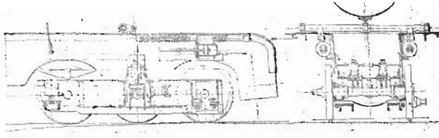
Фиг. 303 и 304. Механизмъ для поднятія и опусканія вспомогательной оси.
