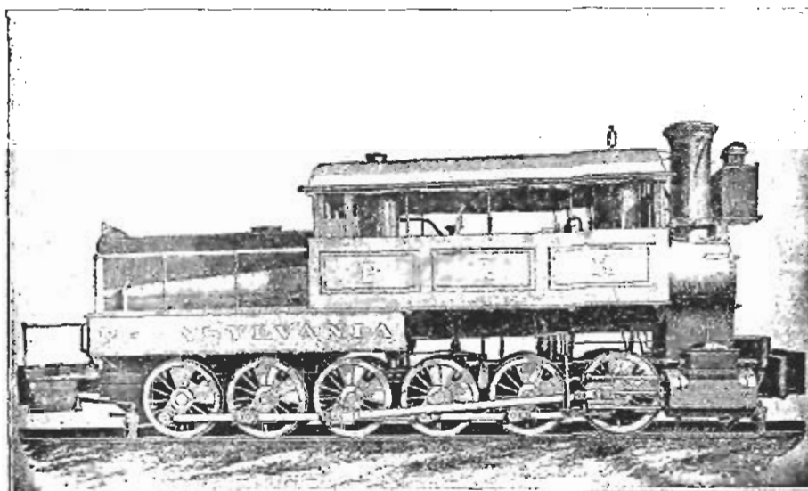
Фиг. 150. Подталкивающій танковый паровозъ ж. д. Филадельфія-Ридингъ. 1865 г.
