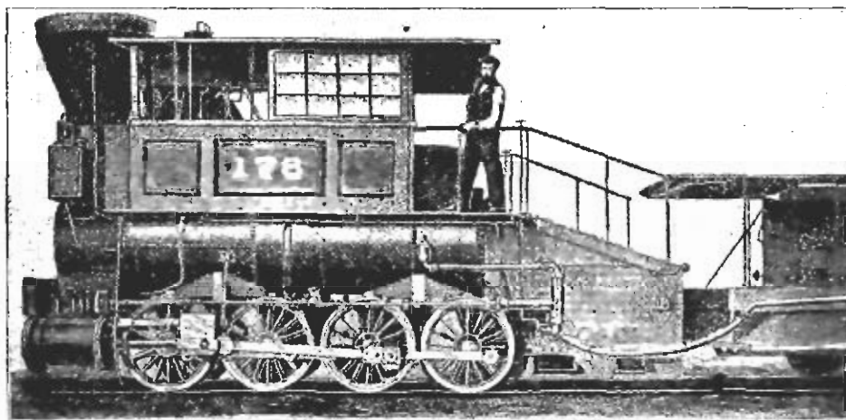
Фиг. 119. Паровозъ „Верблюдъ“ Уайненса, 1852 г.
