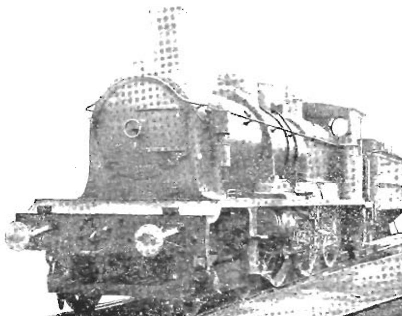
Фиг. 276. 4-хъ цилиндровой compound паровозъ съ 3-ми спаренными осями французской Сѣверной ж. д.
