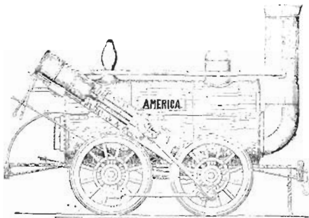
Фиг. 21. Паровозъ „America“, 1828 г.
