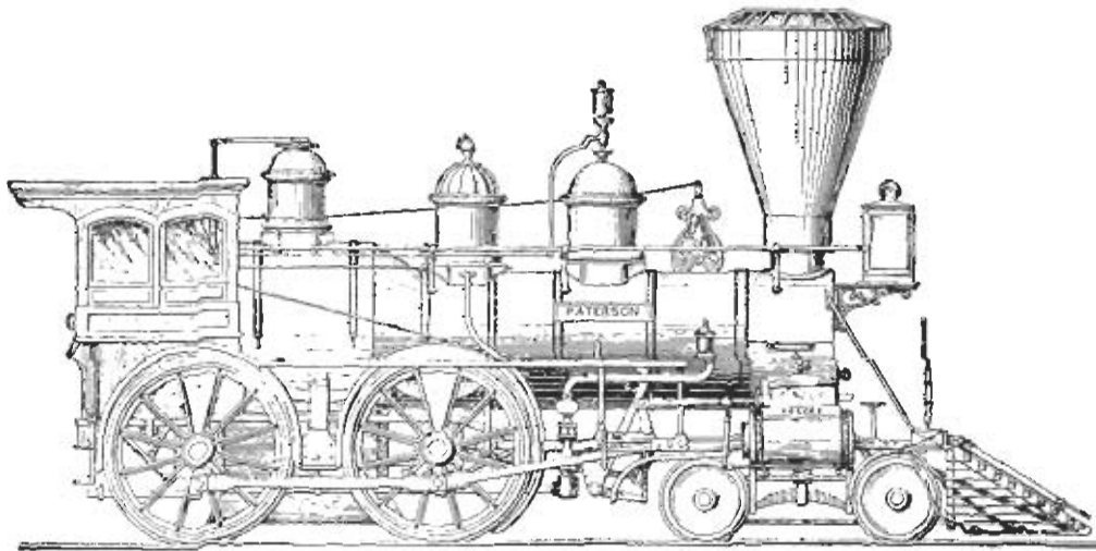
Фиг. 122. Пассажирскій паровозъ „Paterson“. 1853 г.
