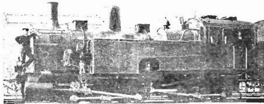
Фиг. 373. Танковый паровозъ системы Нагано's'a 1903 г.
