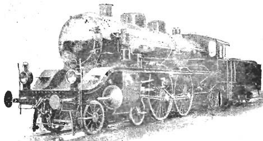
Фиг. 355. Четырех-цилиндровый компаунд-паровозъ Баденскихъ ж. д. 1902 г.
