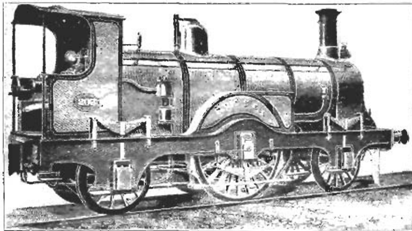
Фиг. 241. Паровозъ жел. дороги Лондонъ, Брайтонъ и Южный берегъ съ парораспределеніемъ Джон.
