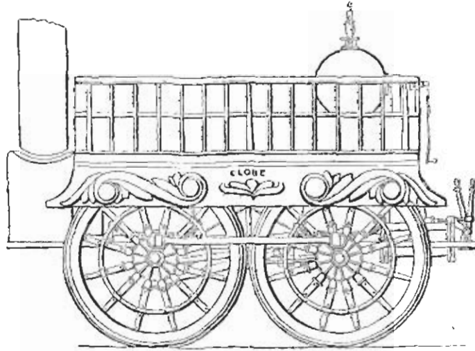
Фиг. 32. Паровозъ „Globe“ Стоктопъ-Дарлингтонской ж. д.
