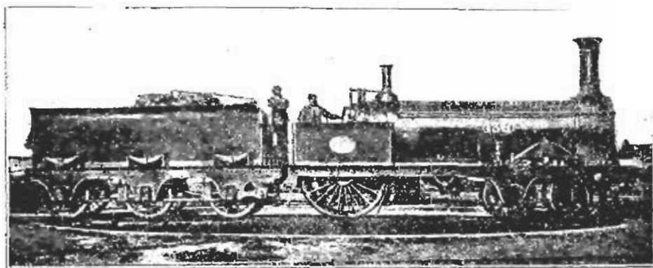
Фиг. 115. Паровозъ „Folkestone“. 1851 г.
