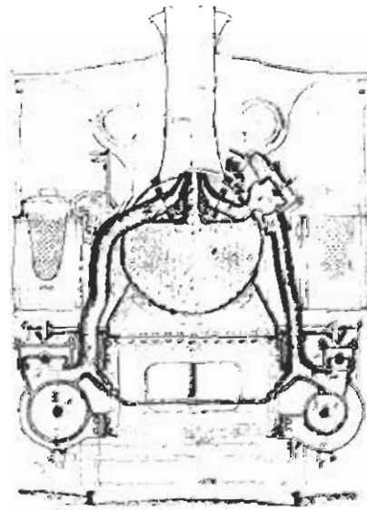
Фиг. 329. Аппаратъ Маллета для пере- мѣны способа работы паровоза.
