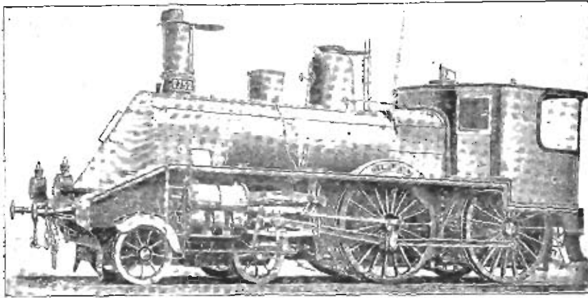
Фиг. 267. Быстроходный паровозъ завода Шнейдера.
