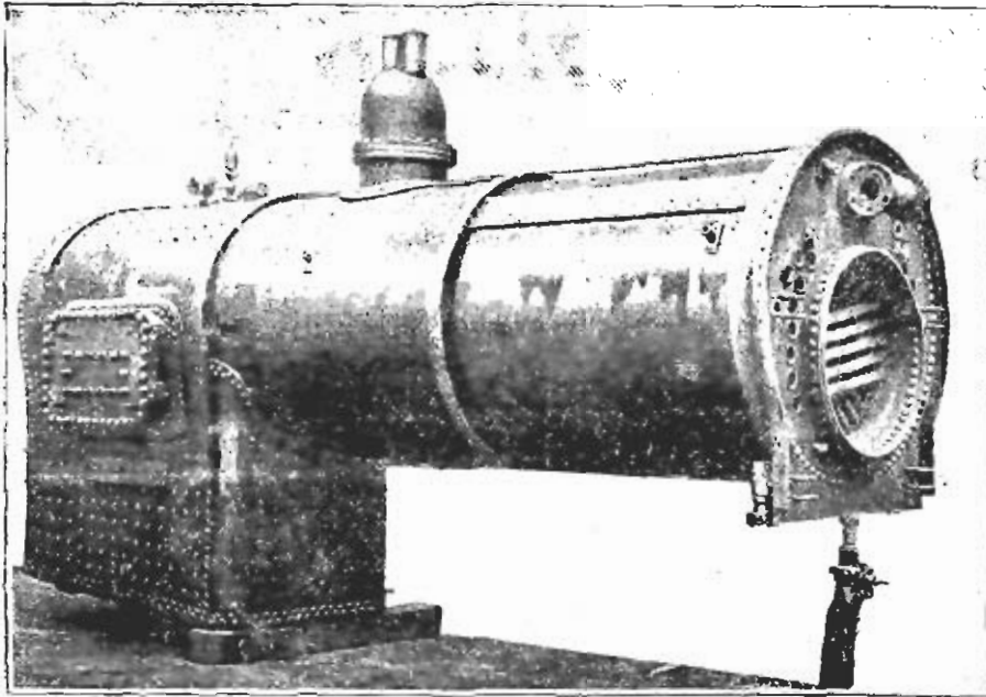
Фиг. 326. Водотрубный паровозный котель. Гаружный видъ.
