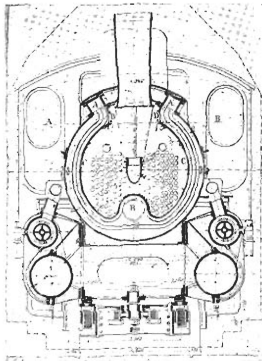
Фиг. 300. Перегриватель. Поперечный разрезь.
