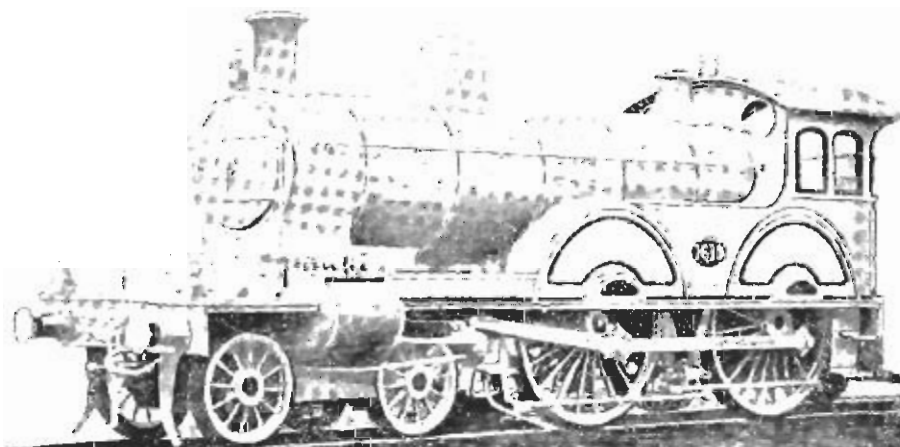
Фиг. 286. 3-хъ цилиндриный compound паровозъ Worsdell'я.
