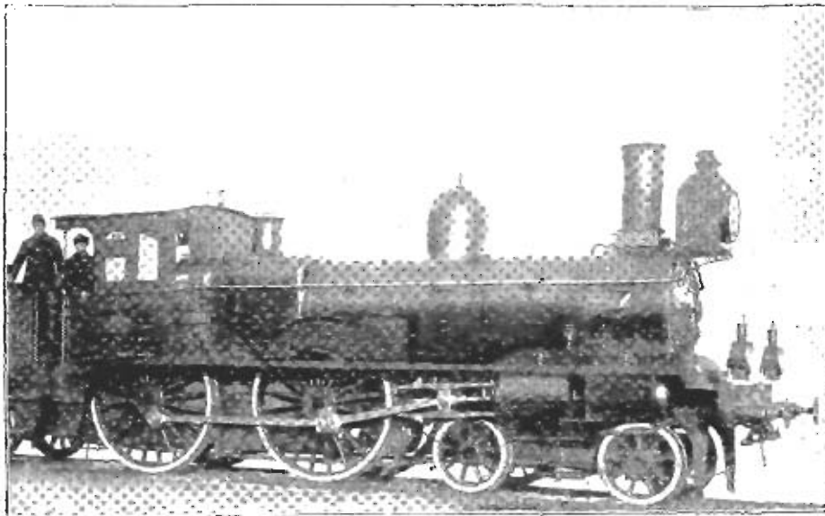
Фиг. 246. Паровозъ гандлемъ компаньей одесскихъ мастерскихъ Юго-западныхъ жел. дорогъ.
