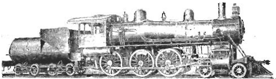
Фиг. 363. Быстроходный 4-хъ цилиндричный компаундъ паровозъ съги желѣзныхъ дор. Plant'a 1902 г.
