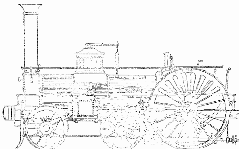
Фиг. 95. Паровозъ „Намур“. Первый паровозъ системы Крамптона.
