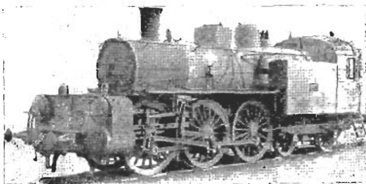
Фиг. 345. Паровозъ-командиръ Южно-итальянской ж. д. завода Борзига: 1901 г.
