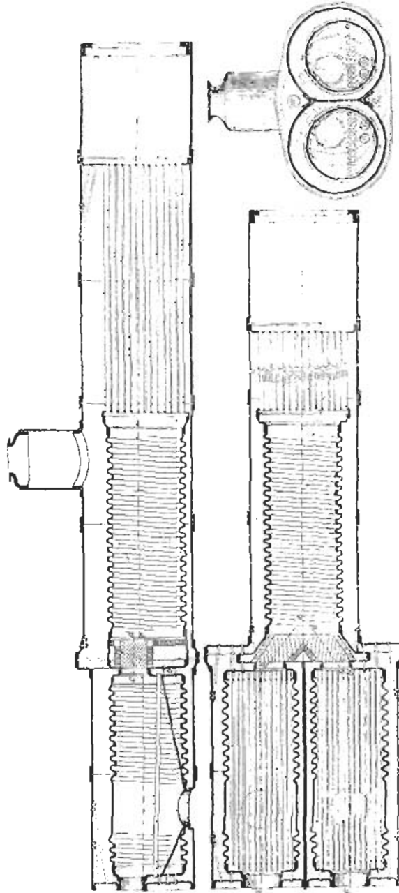
Фиг. 182—184. Котель паровоза Strong'a.
