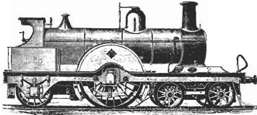
Фиг. 199. Паровозъ системы инженера Samuel'a Johnson'a. 1838 .
