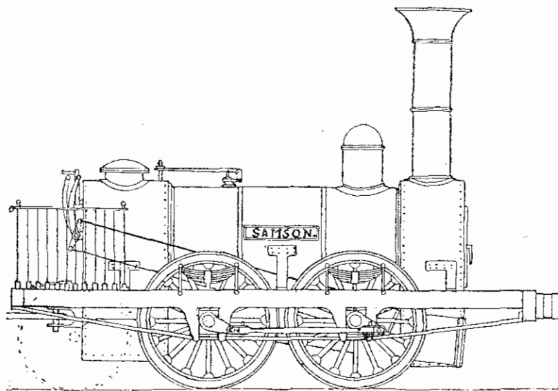
Фиг. 47. Паровозъ „Samson“ Лейстеръ—Суанингтонской ж. д.
