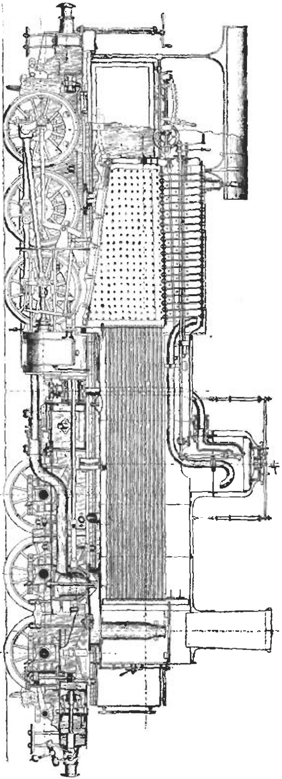
Фиг. 161. Паровозъ системы Meyer'a. 1872 г.
