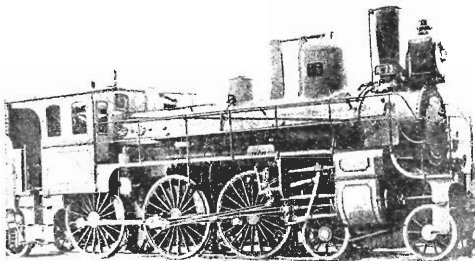
Фиг. 361. Пассажирскій паровозъ компаундъ типа 361 Коломенскаго завода.
