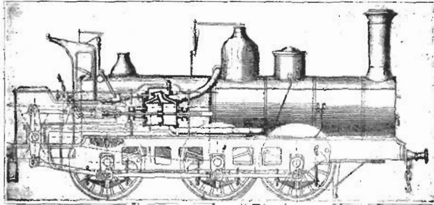
Фиг. 162. Паровозъ Carrel's'a. 1873 г.
