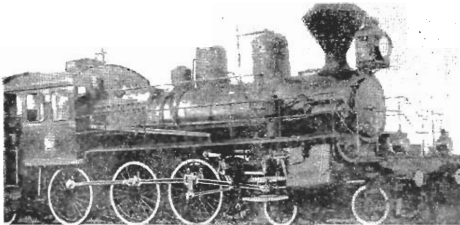
Фиг. 382. Пассажирскій паровозъ компаундъ типа \frac{3}{5} , Восточно-китайской ж. д. построенный Брянскаго завода. 1903 г.
