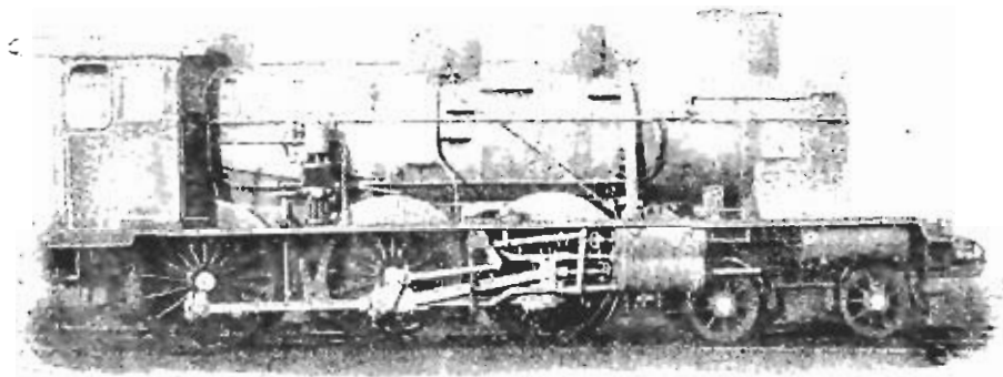
Фиг. 356. Быстроходный компаунд-паровозъ системы Glehn'a. 1902 г.
