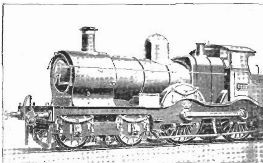
Фиг. 261. Пассажирскій паровозъ Большой западной жел. дороги.
