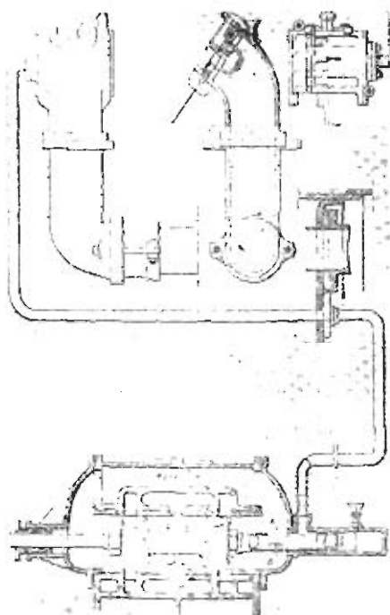
Фиг. 307-309. Расположеніе паропроводныхъ трубы.
