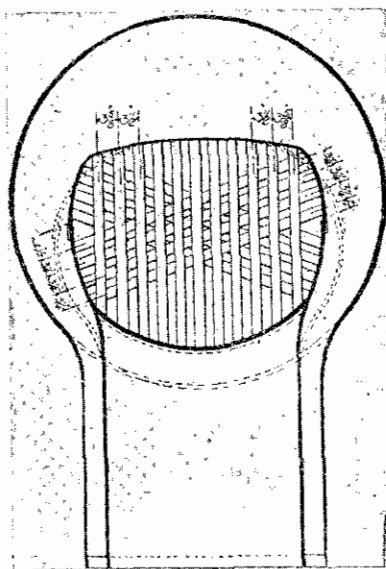
Фиг. 272. Водотрубный котель Перкинса.
