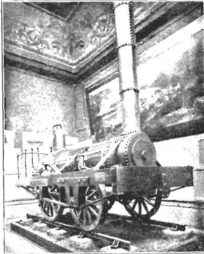
Фиг. 42. Паровоз „Old Ironsides“. Первый паровоз, построенный Балдвиномъ, 1832 г.
