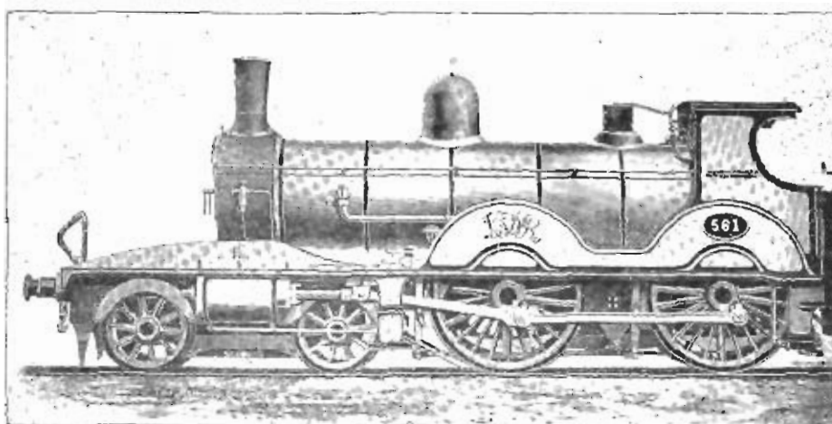
Фиг. 217. Пассажирскій паровозъ Adams'a.
