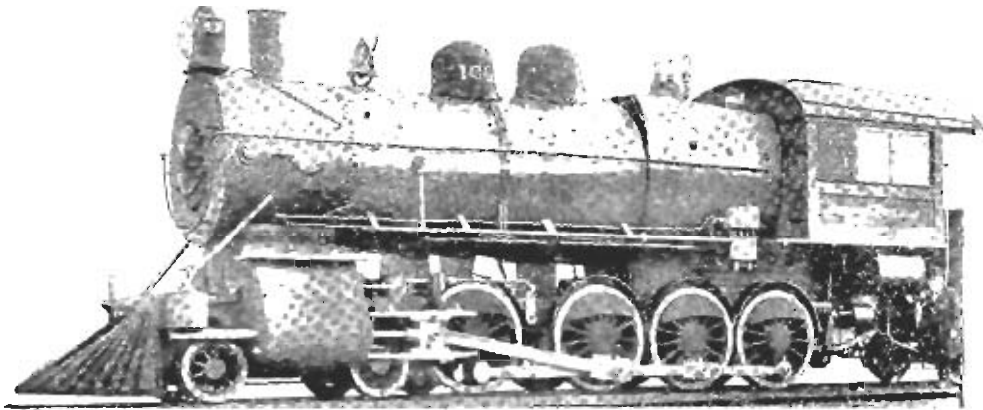
Фиг. 273. Паровозъ типа „мастодонтъ“ завода Брукса.
