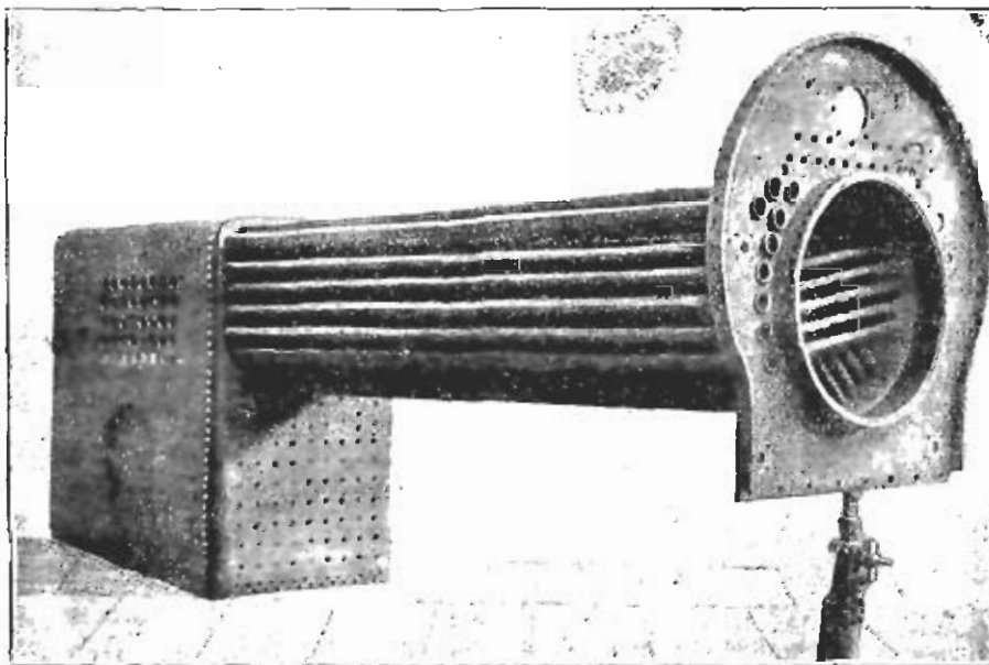
Фиг. 327. Водотрубный паровозный котель. Труба, передняя трубная доска и огневая коробка.
