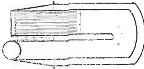
Фиг. 26. Котель паровоза „Sanspareil“.
