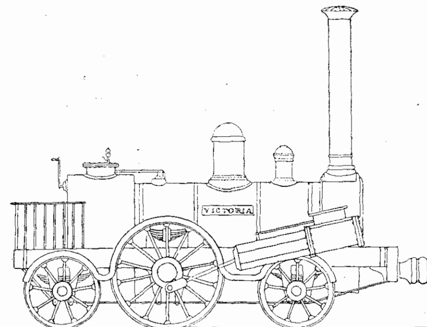
Фиг. 75. Паровозъ „Victoria“. 1838 г.
