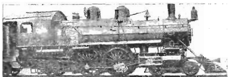
Фиг. 386. Пассажирскій 4-цилиндровый компаундъ паровозъ Atchison, Toroka & Santa Fé ж. д. 1903 г.
