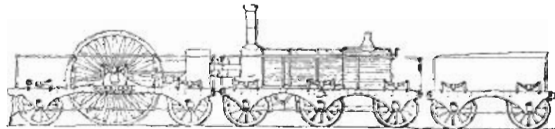
Фиг. 71. Паровозъ Гаррисона „Ураганъ“.
