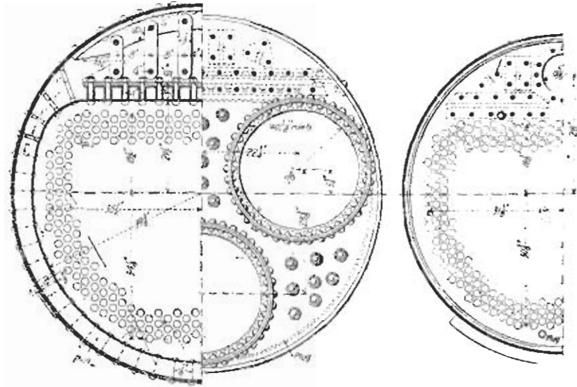
Фиг. 392 и 393. Поперечный разрѣзъ тендера.
