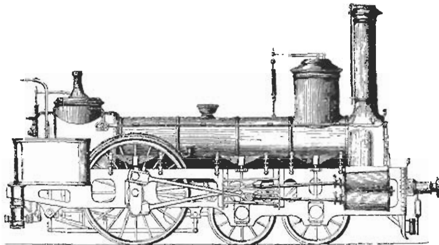
Фиг. 141. Паровозъ „Duplex“ Гасвеля.
