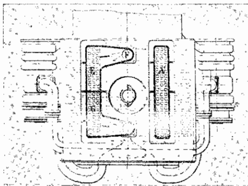
Фиг. 301. Перегрѣватель. Плавъ.
