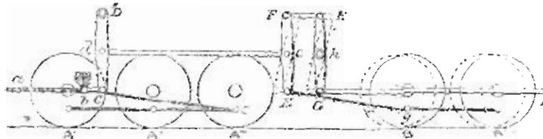
Фиг. 374. Устройство передаточнаго механизма.
