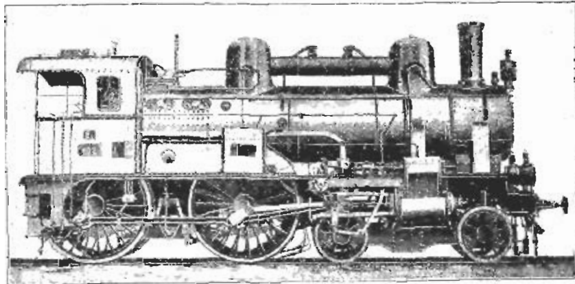
Фиг. 263. Пассажирскій паровозъ компаніи австрійскихъ жел. дорогъ
