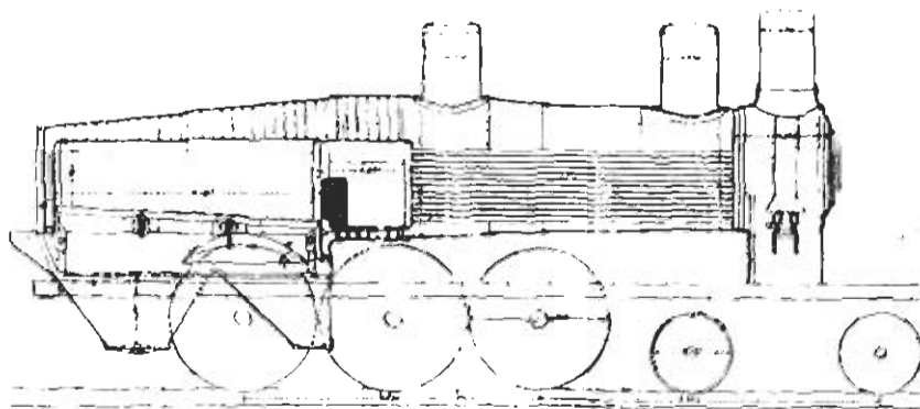
Фиг. 236. Топка системы Wooten.
