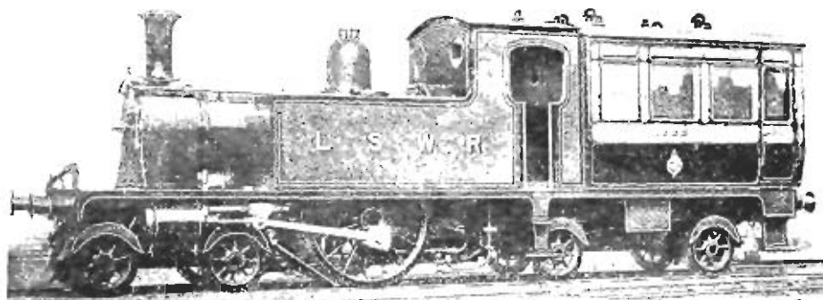
Фиг. 292. Паровозъ-вагонъ Лондонъ-Юго Западной ж. д.
