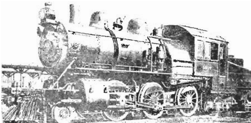
Фиг. 365. Пассажирскій паровозъ Нью-Йоркъ-Центральной ж. д. 1902 г.
