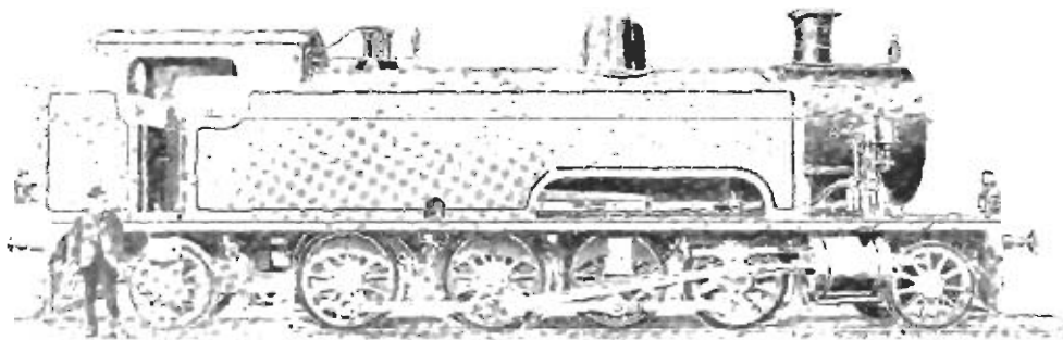
Фиг. 277. Танковый паровозъ завода Neilson'a.
