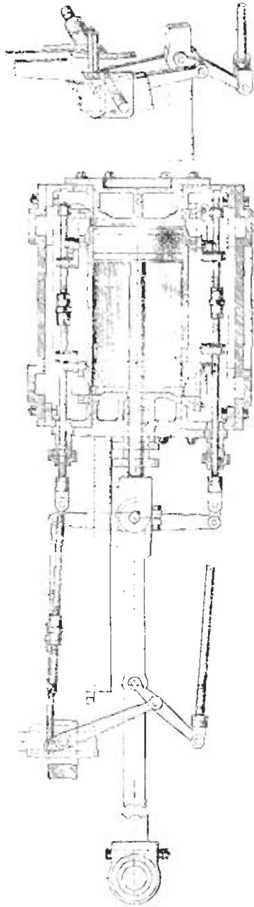
Фиг. 185—186. Парораспределение паровоза Strang'a.
