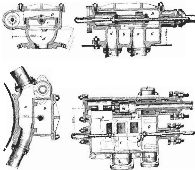
Фиг. 330-333. Автоматическій расширитель Маллета.
