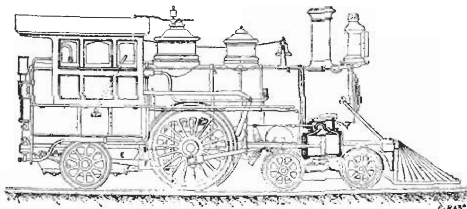
Фиг. 170. Паровозъ завода Бальдвина съ переменной нагрузкой ведущей осю.
